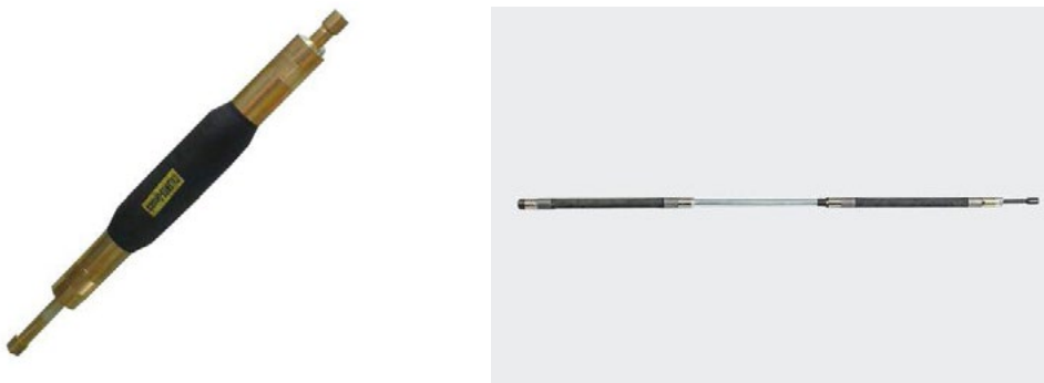
Fig.4: Obturador inflable simple (izquierda) (© italswiss.com) y obturador doble (derecha) (© desoi.it)
